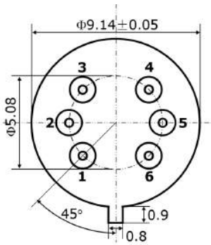
TO39 schematic
